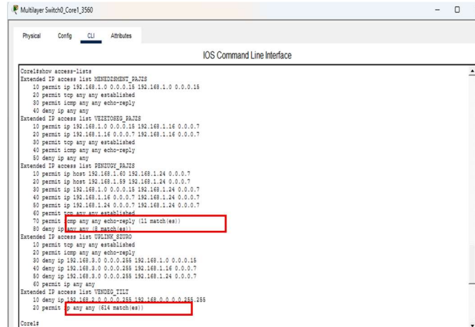
M2-5. ábra – ACL találati statisztikák Forrás: Saját készítésű képernyőkép
